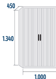
ARMP-13/1 COD: 13410 3 plateaux
