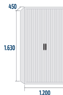
ARMP-16/2 COD: 16312 3 plateaux
