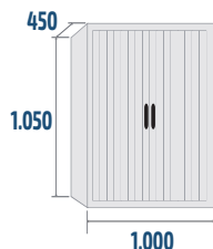
ARMP-10/1 COD: 10510 2 plateaux
