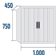
ARMP-07/1 COD: 07510 1 plateau
