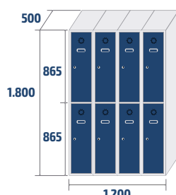
ECOT-30/4 COD: 83014 61,4kg · 1,08m 3
