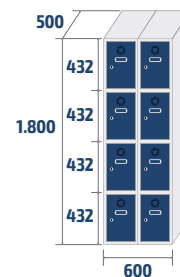
ECOC-30/2 COD: 83022 38,6kg · 0,54m 3
