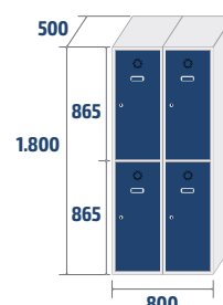
ECOT-40/2 COD: 84012 41kg · 0,72m 3
