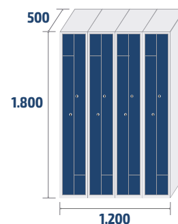
ECOL-30/4 COD: 35304 79,8kg · 1,08m 3
