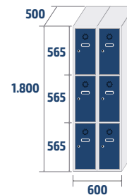
ECOM-30/2 COD: 83032 36,4kg · 0,54m 3
